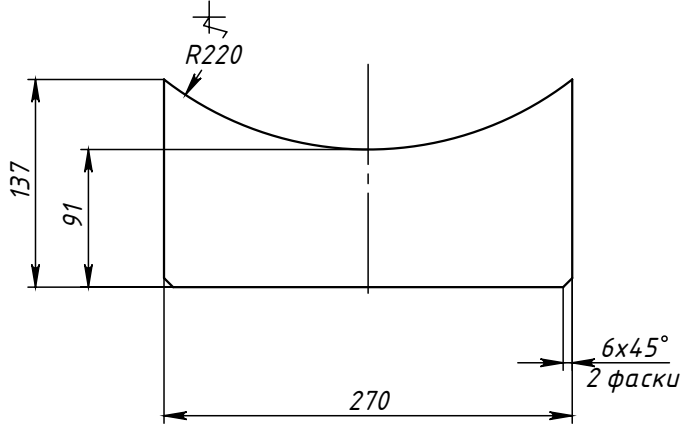
Поз.3 (Ребро)
